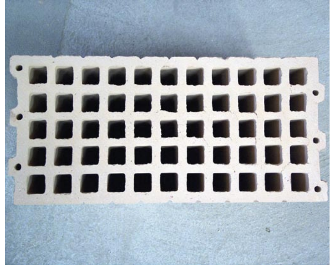
Bilder 2/3: Beispiele für Hochlochziegel mit in Wandlängsrichtung durchgehenden Innenstegen für einschalige Außenwände
